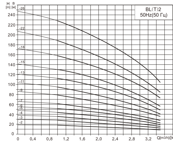
■ Performance curves(Кривые производительности)
