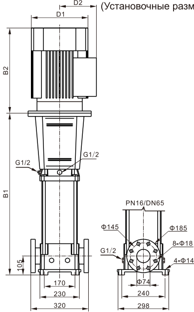
Performance parameters and dimensions weight(Параметры производительности и объемный вес)
