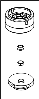
Выпускная камера
