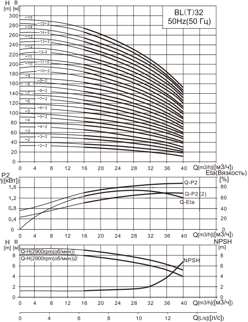
Performance parameters and dimensions weight(Параметры производительности и объемный вес)
