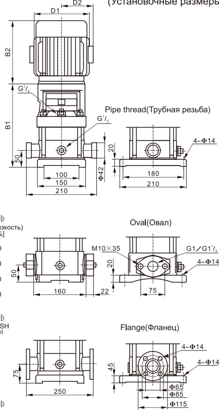
■ Installation dimensions (Установочные размеры)
