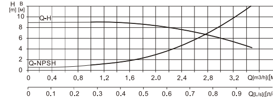
■ Performance parameters and dimensions weight(Параметры производительности и объемный вес)
